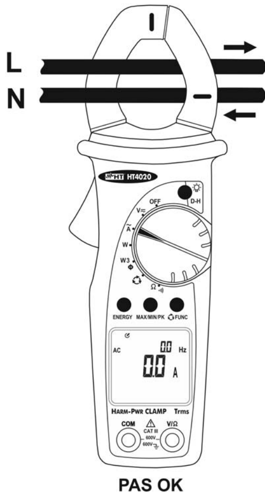
Fig. 8 : Mesure de courant AC
