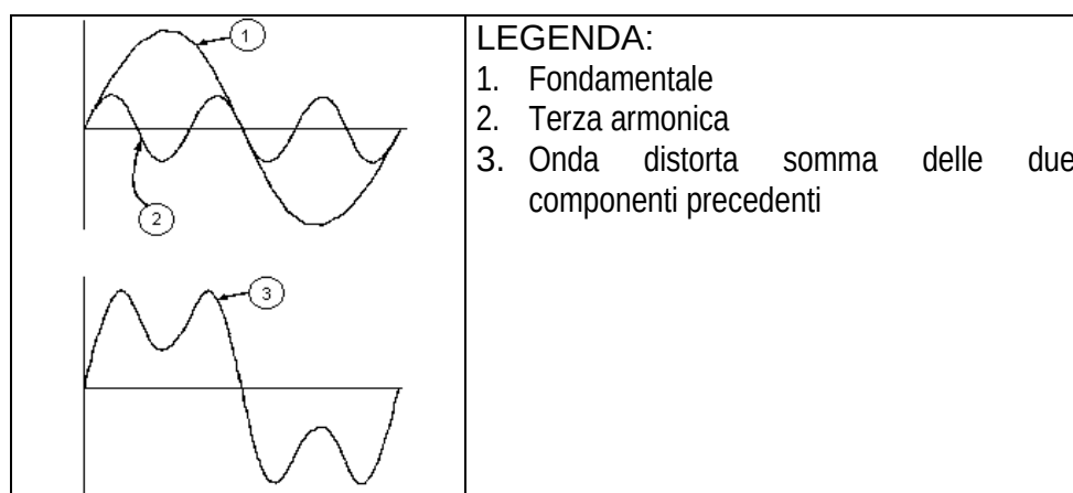
Effetto della somma di 2 frequenze multiple.
